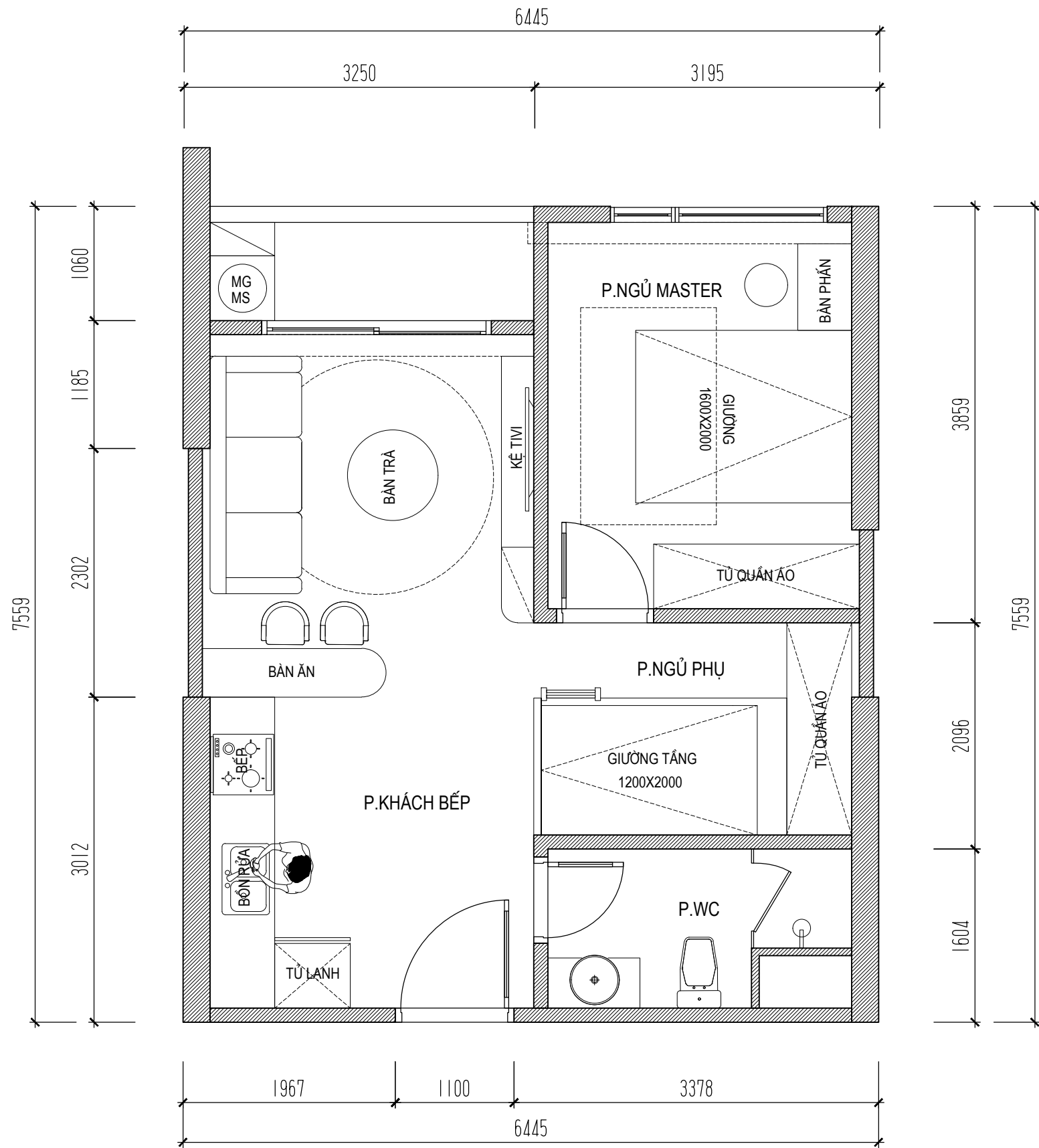
PHƯƠNG ÁN II BỐ TRÍ MẶT BẰNG CĂN HỘ
