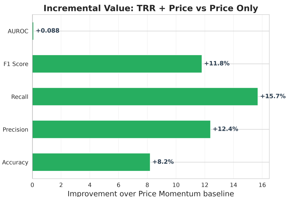
Figure 9: Giá trị gia tăng cận biên của tín hiệu LLM khi được so sánh trực diện với đà giá thuần túy (Price momentum).
