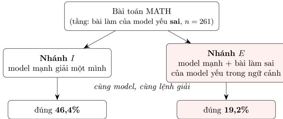
Hình 1: Thí nghiệm tác động artifact — cho model mạnh xem bài làm của model yếu (thiết kế chốt trước, MATH-500): hai nhánh chỉ khác nhau ở việc ngữ cảnh có kèm bài làm sai của model yếu hay không. Chênh lệch -27,2 điểm ( p \approx 0 ) là nguồn thiệt hại chính của các giao thức cho model sửa bài của nhau (§5.9).
