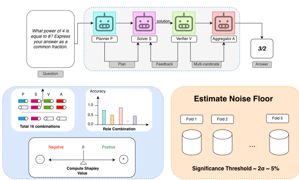
Hình 2: Sơ đồ pipeline bốn vai trò, 16 tổ hợp bật/tắt để tính giá trị Shapley, và quy trình ước lượng nhiễu qua 5 fold.
