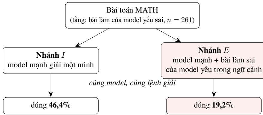
Hình 1: Thí nghiệm tác động artifact — cho model mạnh xem bài làm của model yếu (thiết kế chốt trước, MATH-500): hai nhánh chỉ khác nhau ở việc ngữ cảnh có kèm bài làm sai của model yếu hay không. Chênh lệch -27,2 điểm ( p \approx 0 ) là nguồn thiệt hại chính của các giao thức cho model sửa bài của nhau (§5.9).
