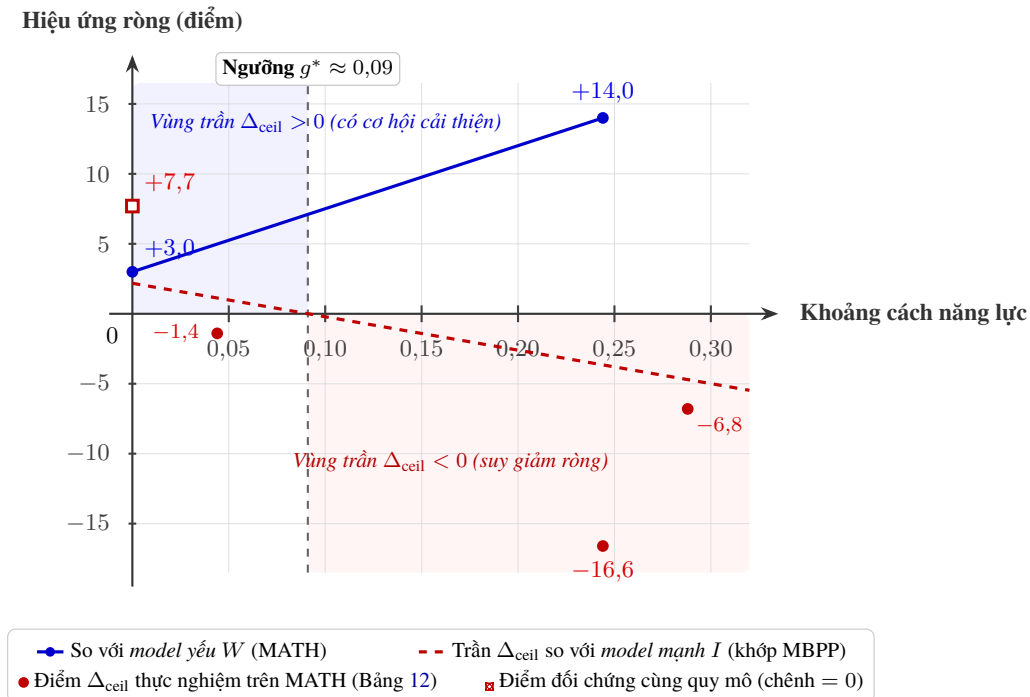
Hình 4: Nghịch lý mốc tham chiếu. Trục hoành là khoảng cách năng lực: hiệu ứng đo so với model yếu W (đường xanh liền) tăng mạnh do cộng hưởng năng lực; trong khi trần giá trị ròng \Delta_{\text{ceil}} so với model mạnh I (đường đỏ đứt: khớp trên 15 cặp MBPP; các chấm đỏ: 3 điểm đo MATH) suy giảm nhanh và đổi dấu sang âm khi vượt ngưỡng tới hạn g^* \approx 0,09 do tổn thất phơi nhiễm L áp đảo cơ hội cải thiện G .
