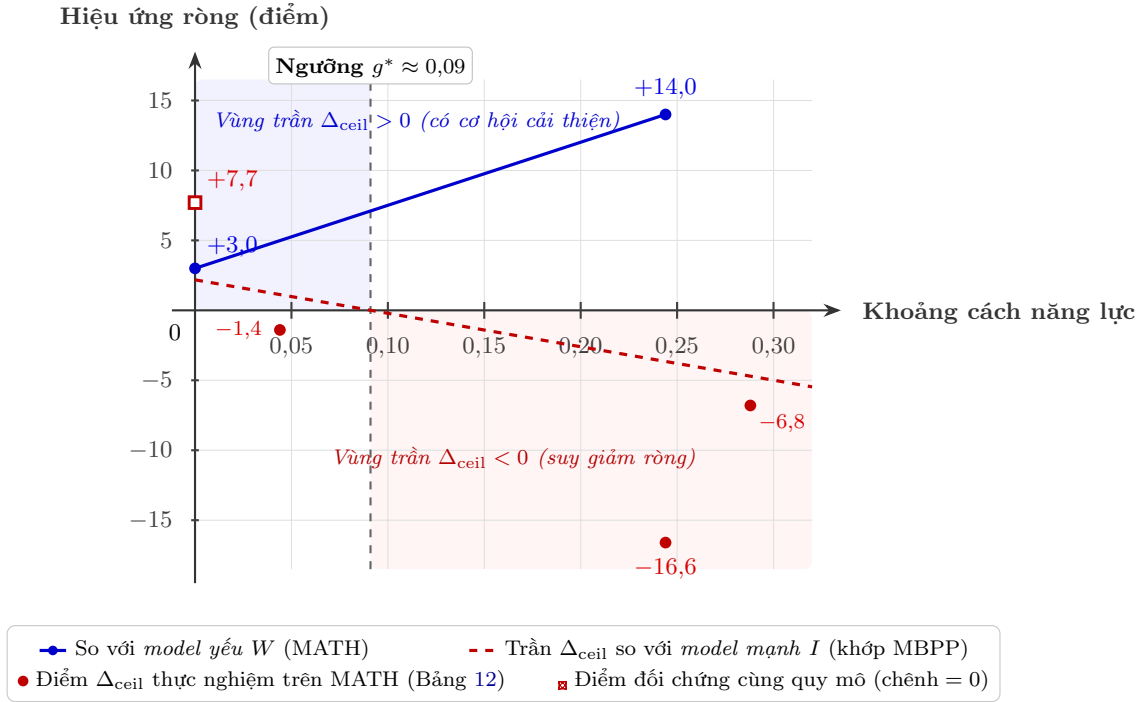
Hình 4: Hai mốc so sánh, hai chiều biến thiên. Trục hoành là khoảng cách năng lực: hiệu ứng đo so với model yếu W (đường xanh liền) tăng mạnh do cộng hưởng năng lực; trong khi trần giá trị ròng \Delta_{\text{ceil}} so với model mạnh I (đường đỏ đứt: khớp trên 15 cặp MBPP; các chấm đỏ: 3 điểm đo MATH) suy giảm nhanh và đổi dấu sang âm khi vượt ngưỡng tới hạn g^* \approx 0,09 do tổn thất phối nhiệm L áp đảo cơ hội cải thiện G .
