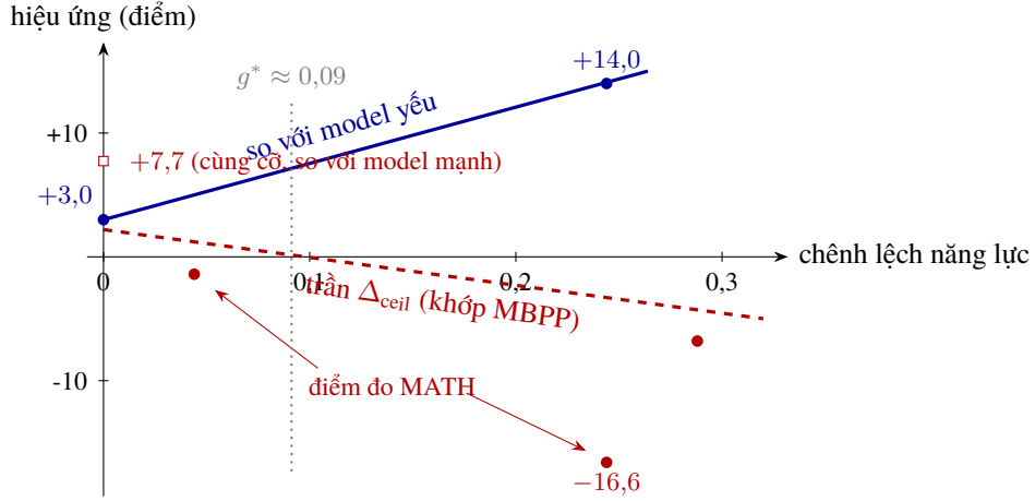
Hình 4: Nghịch lý móc so sánh. Cùng trục hoành là chênh lệch năng lực; hiệu ứng đo so với model yếu (đường liền; hai điểm đo MATH) tăng; giá trị so với model mạnh (đường đứt: khớp trên 15 cặp MBPP; chấm đỏ: ba điểm đo MATH của Bảng 12; ô vuông: điểm +7,7 tại chênh 0) giảm và âm sau g^* . Hình vẽ đúng số liệu nhưng nổi hai thiết lập khác nhau — xem Bảng 10 trước khi so hai đường theo trục tung.
