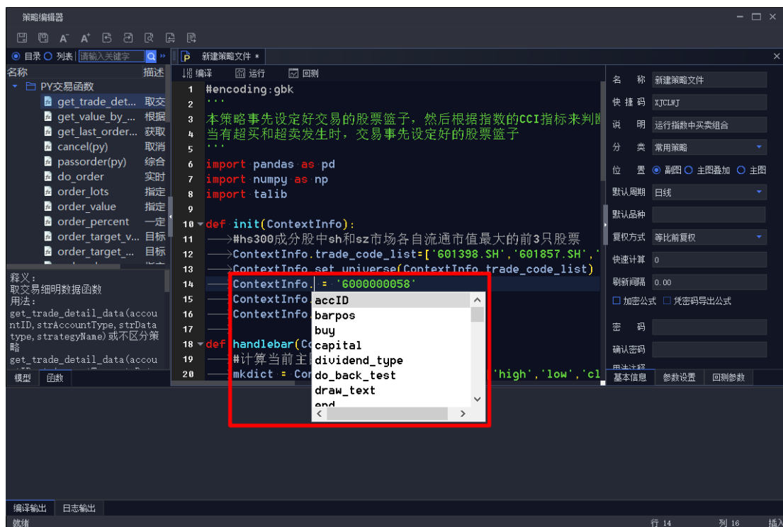
图 23 模型编辑器—代码补全
