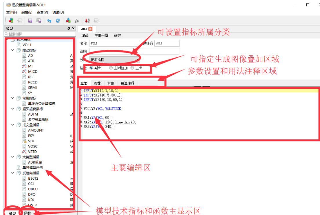
图 49 VBA 模型编辑功能区介绍
