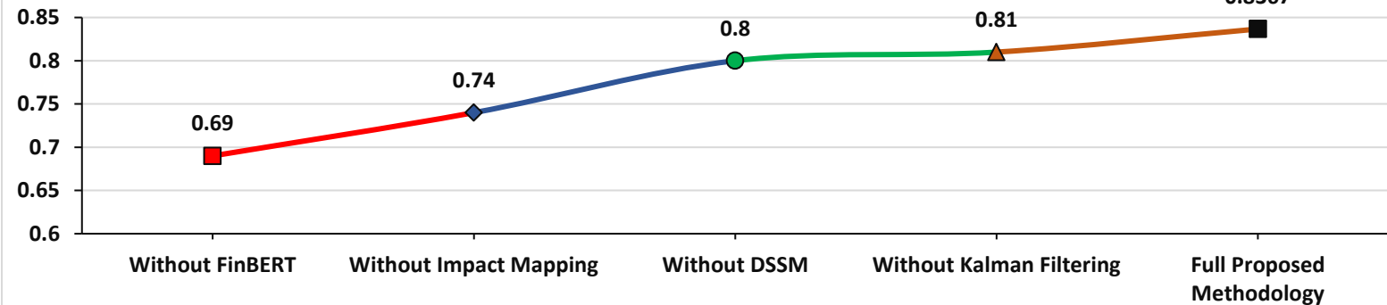
R2
