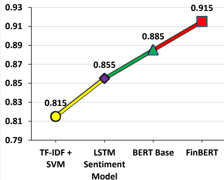
F1 Score
