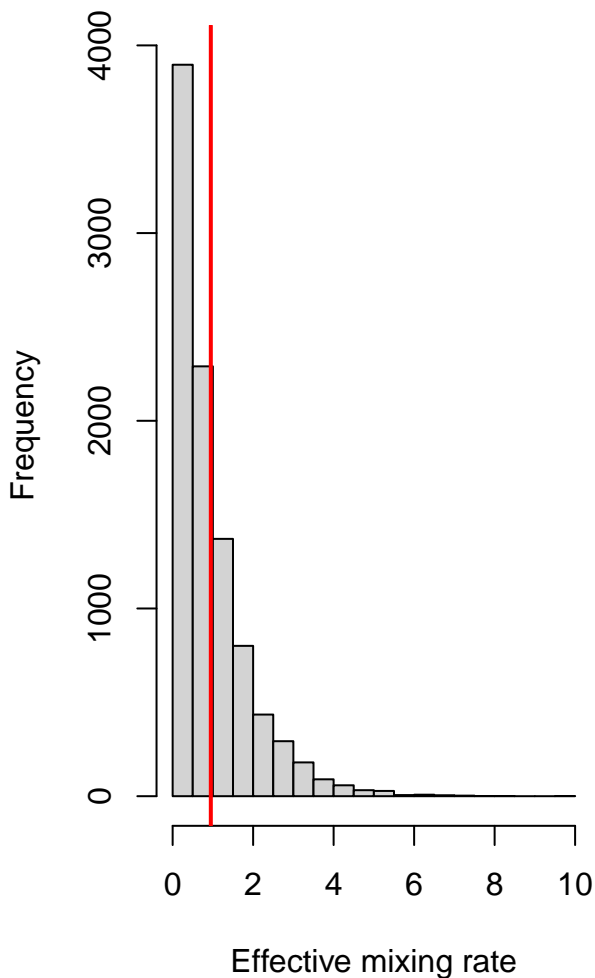
Susceptible
