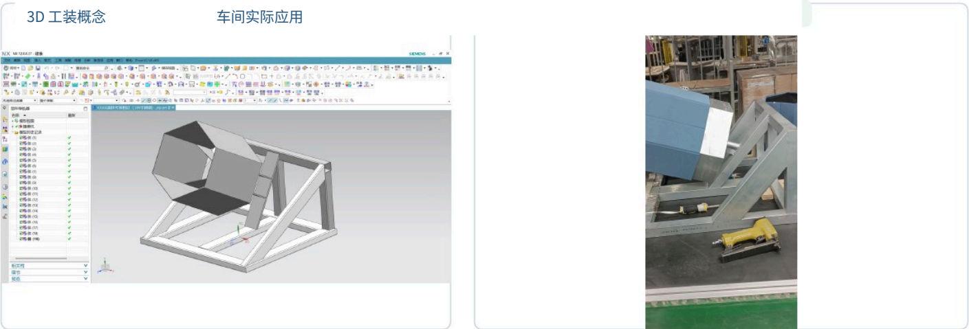
定位/翻转工装：另一套 NX 概念与已制成并用于生产现场的工装相对应。同一时期还保留多套工装夹具的实物照片。
