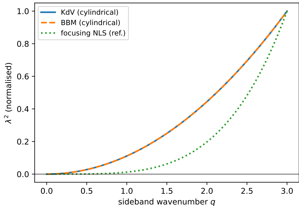
\lambda^2 > 0 : stable; \lambda^2 < 0 : MI band
