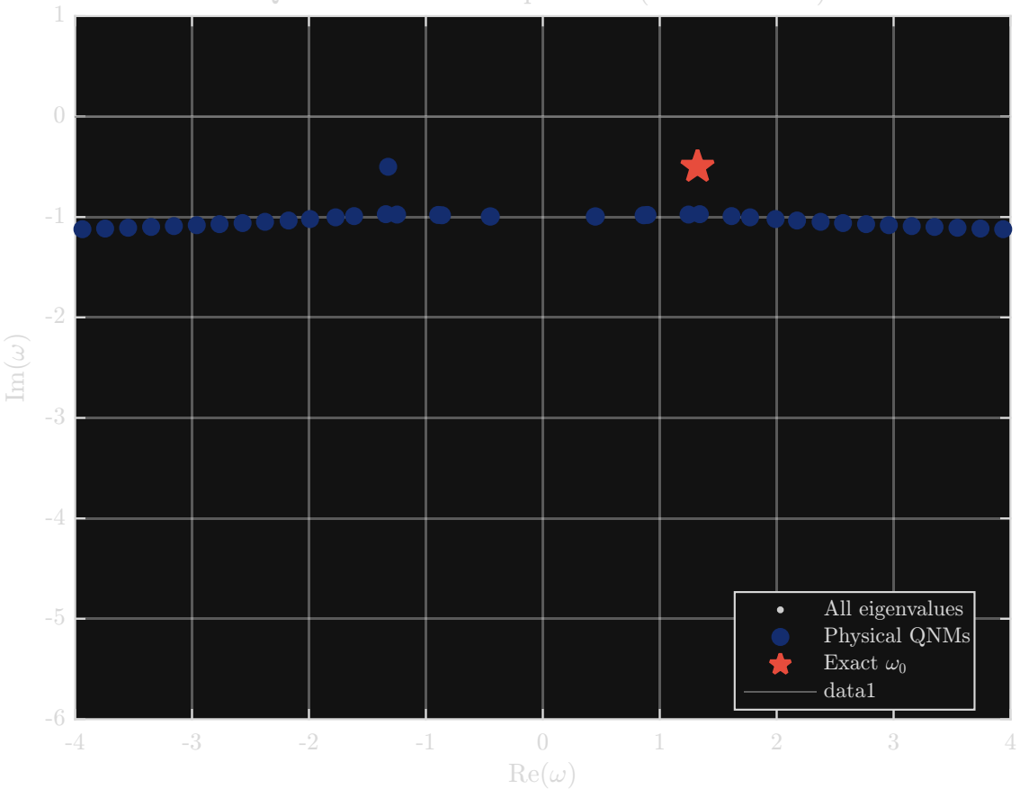
Quasinormal Mode Spectrum (Pöschl–Teller)
