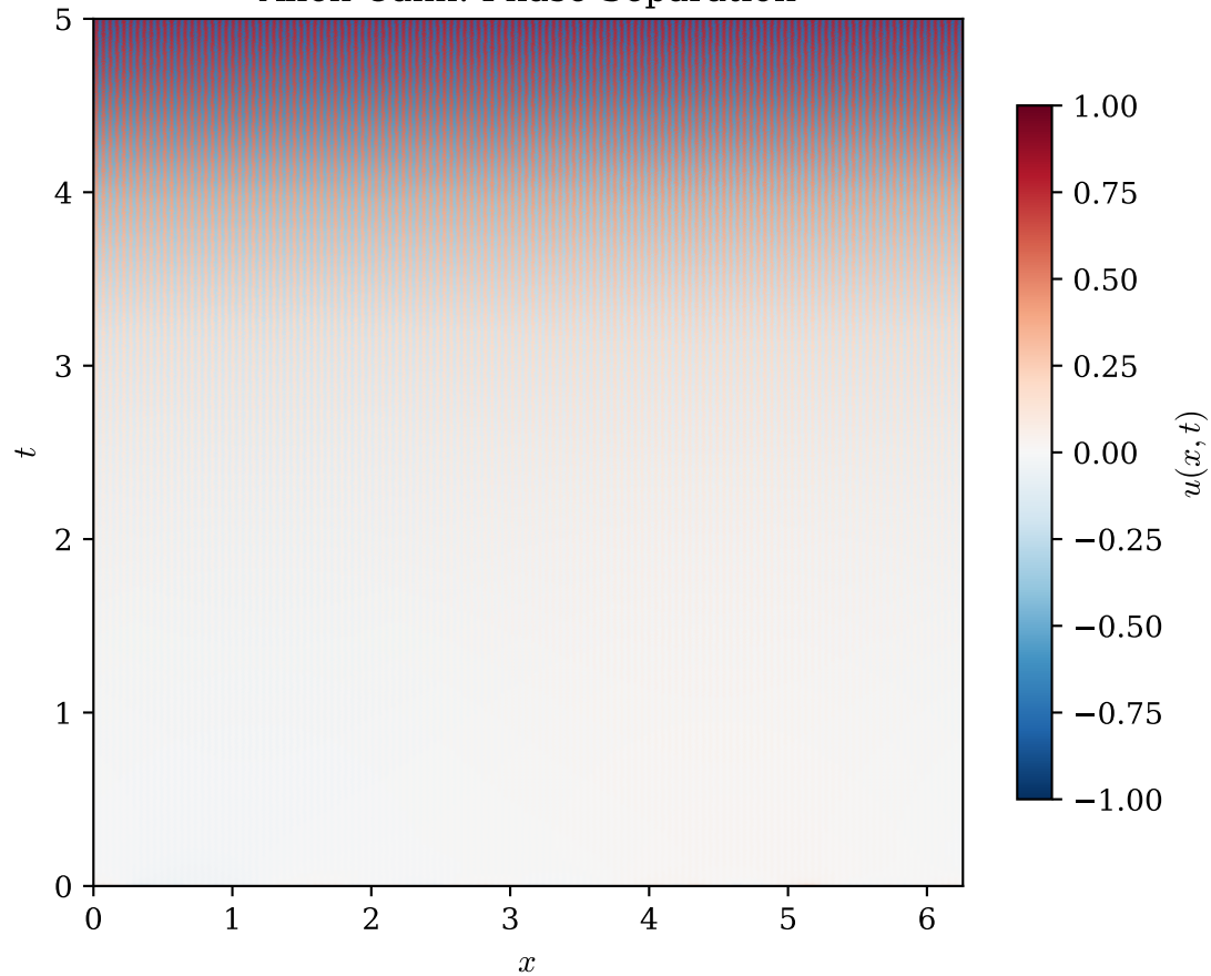
Allen-Cahn: Phase Separation
