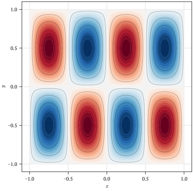
(d) (2, 4) Dirichlet eigenmode shape
