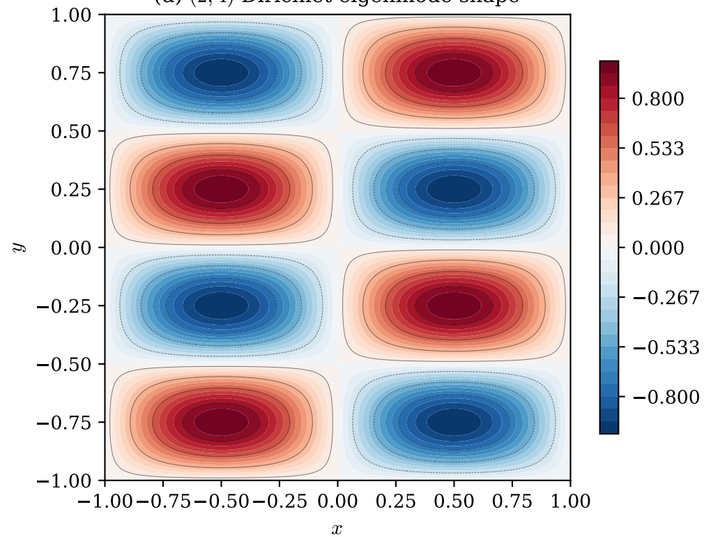
(d) (2, 4) Dirichlet eigenmode shape
