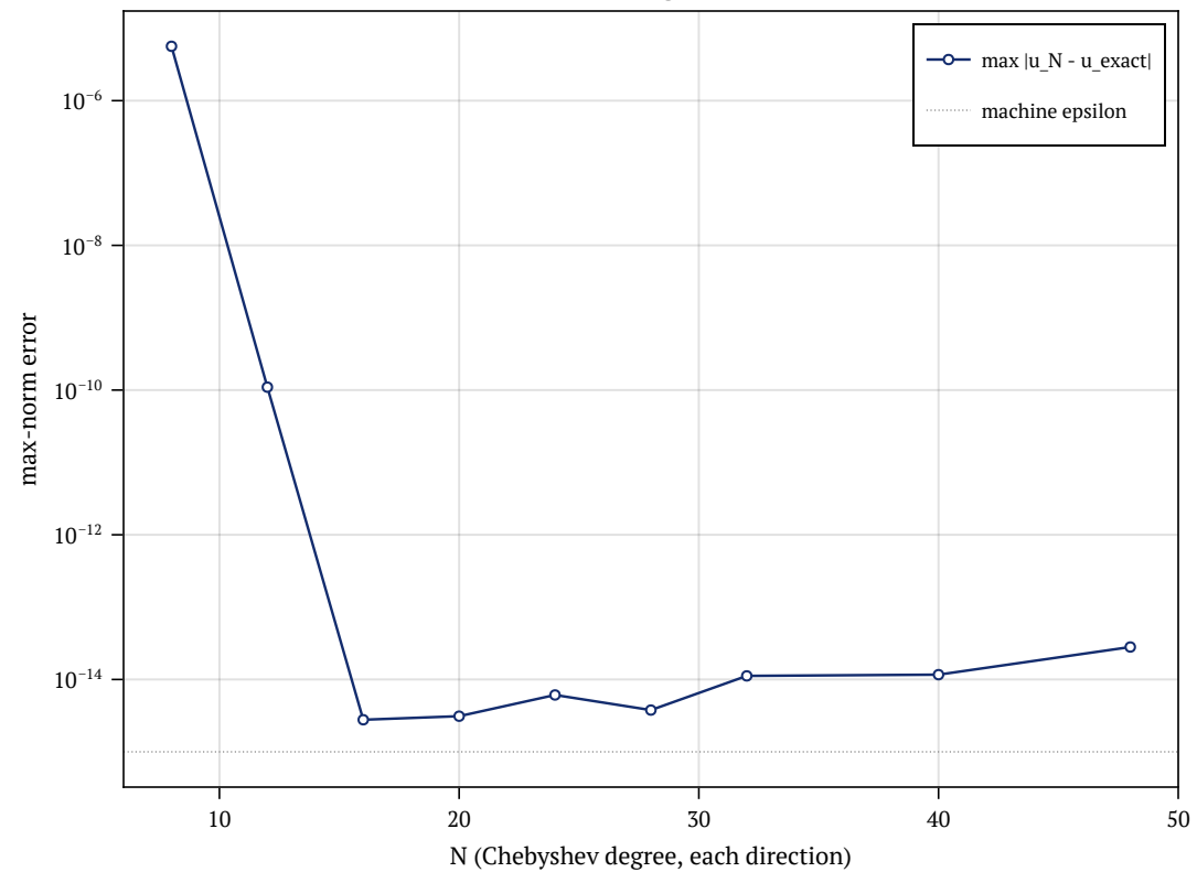
(d) spectral convergence: error vs N
