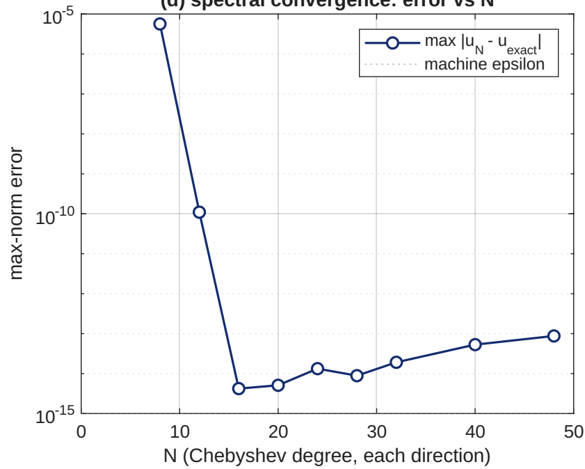
(d) spectral convergence: error vs N
