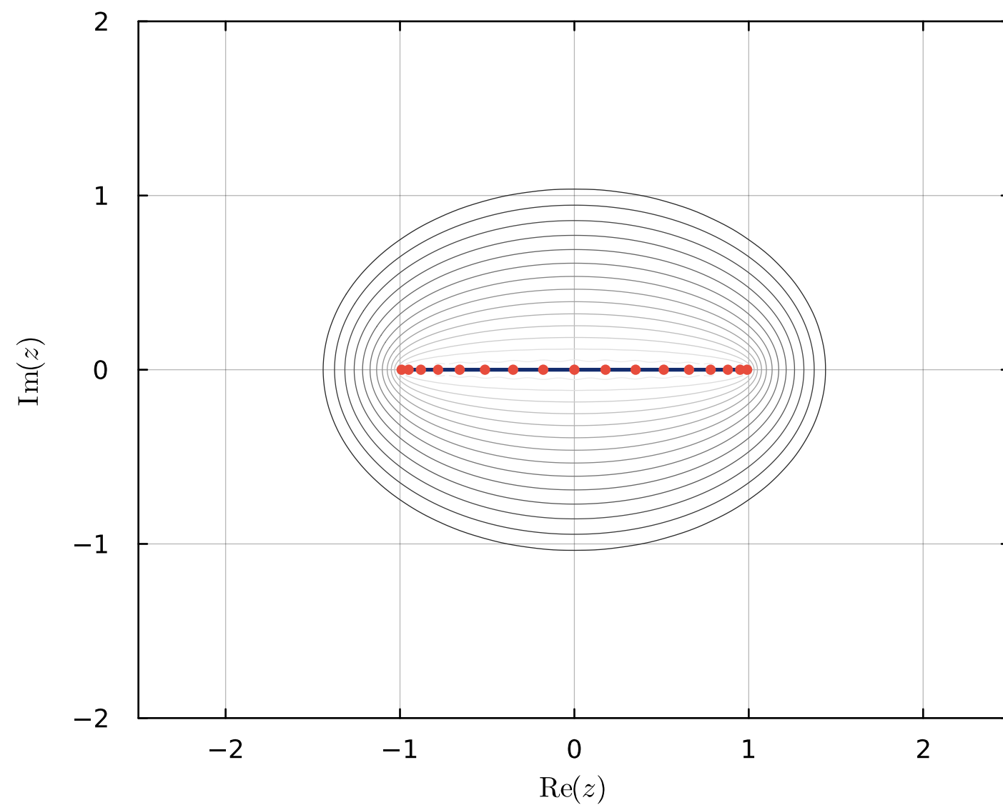
(d) convergence on \int_{-1}^1 dx/(1+16x^2)
