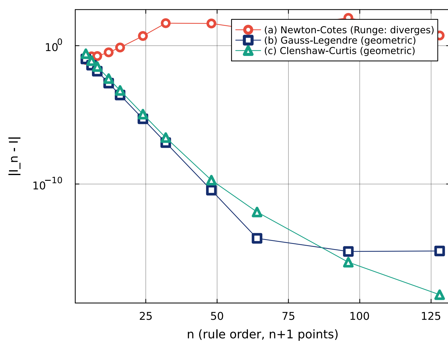
(d) convergence on \int_{-1}^1 dx/(1+16x^2)
