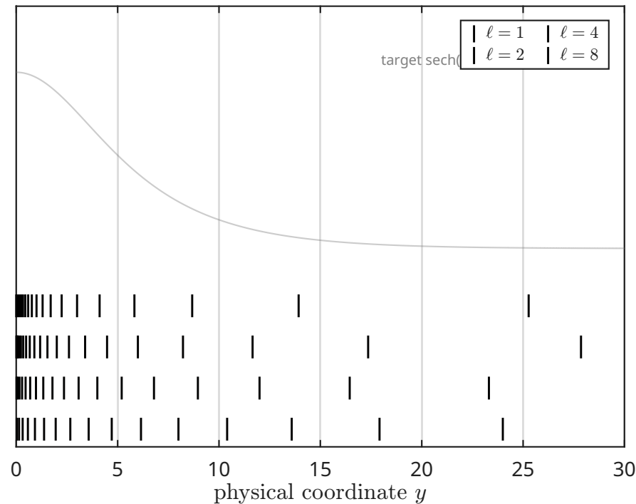
(d) coefficient diagnostic: \text{TL}_n expansion of \text{sech}(y)
