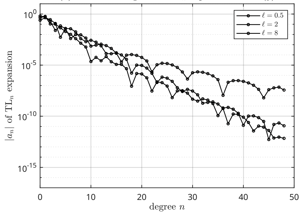
(d) coefficient diagnostic: \text{TL}_n expansion of \text{sech}(y)
