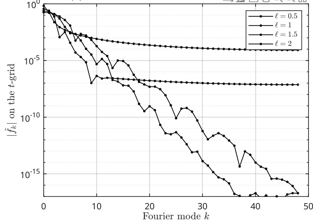
(d) Fourier-in- t coefficients of \text{sech}(y)
