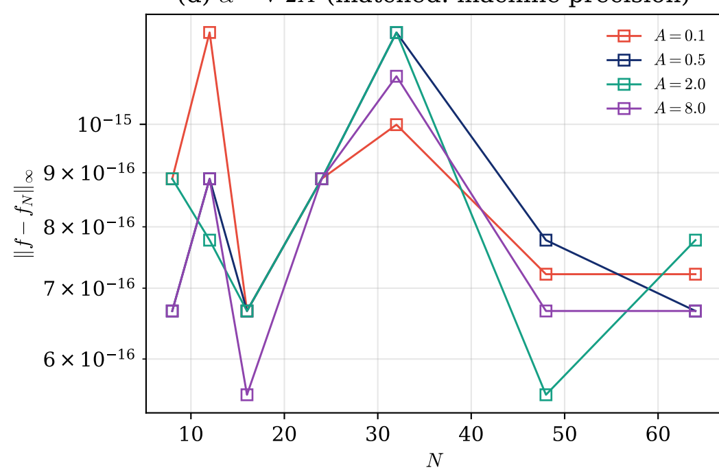
(d) \alpha=\sqrt{2A} (matched: machine precision)
