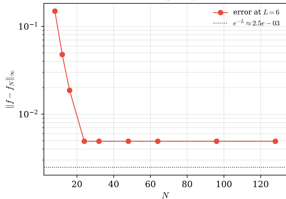
(a) Fix L , vary N : plateau
