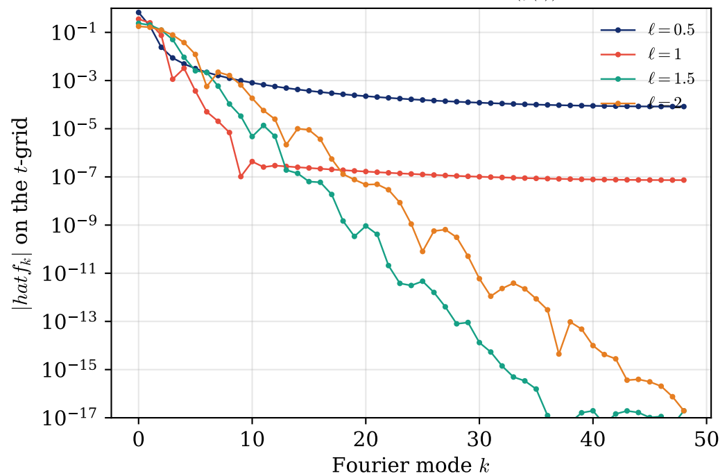
(d) Fourier-in- t coefficients of \text{sech}(y(t)) , N = 96
