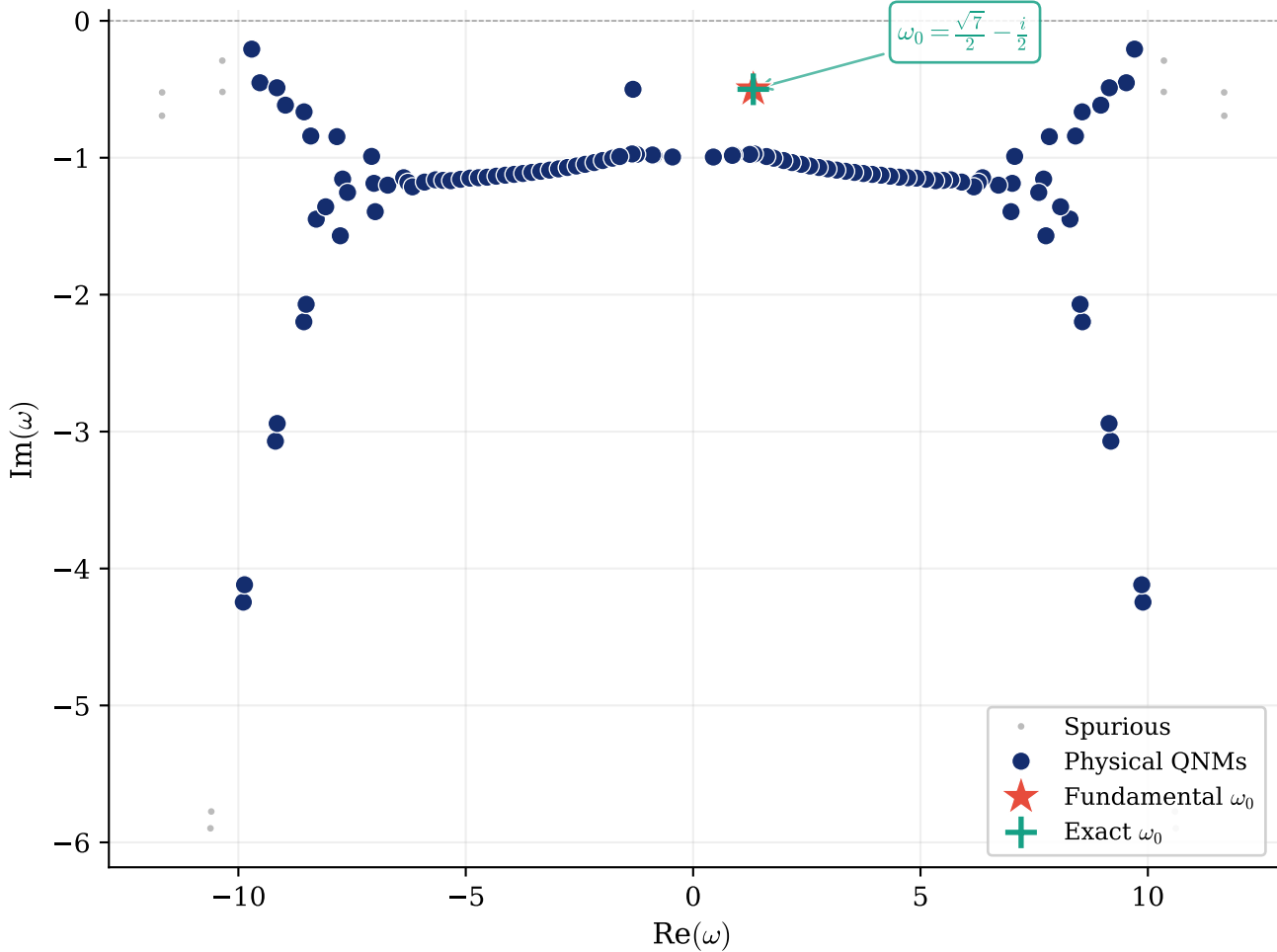
QNM Spectrum: Pöschl-Teller Potential ( V_0 = 2 )
