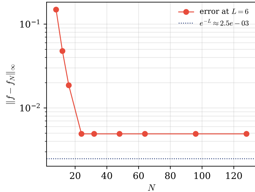
(a) Fix L , vary N : plateau
