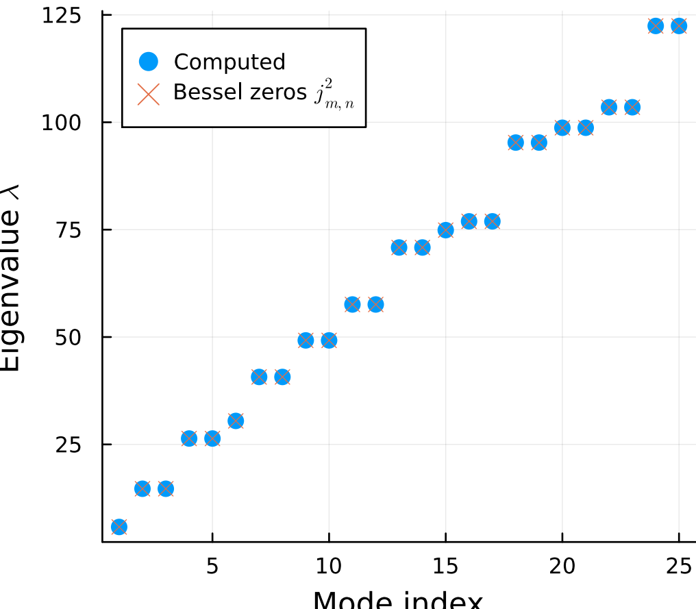
Eigenvalue comparison
