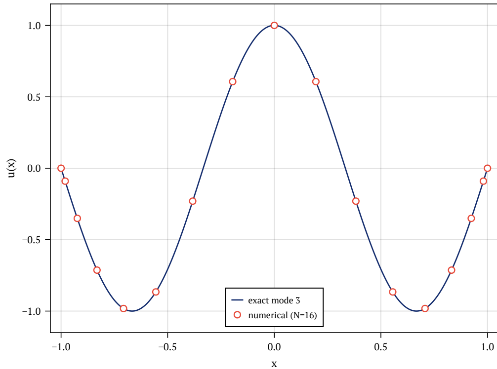
mode j=3: \lambda_{\text{num}}=22.2066 , \lambda_{\text{exact}}=22.2066
