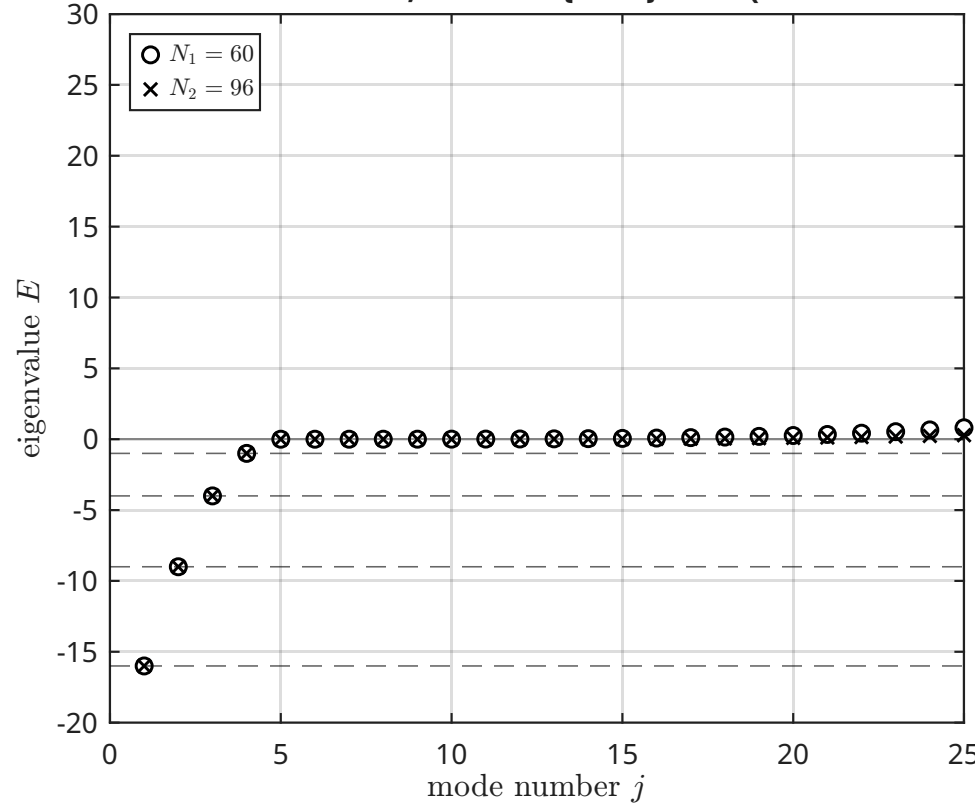
Pöschl-Teller V = -4 \cdot 5 \cdot \mathrm{sech}^2 x (exact: 4 boundstates)
