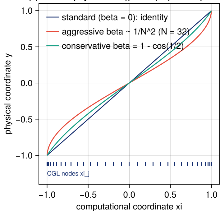
(a) KTE map y = \arcsin((1-\beta)x)/\arcsin(1-\beta)
