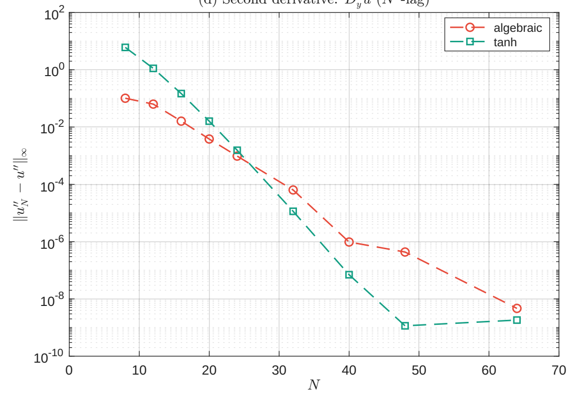
(d) Second derivative: D_y^2 u ( N^2 -lag)
