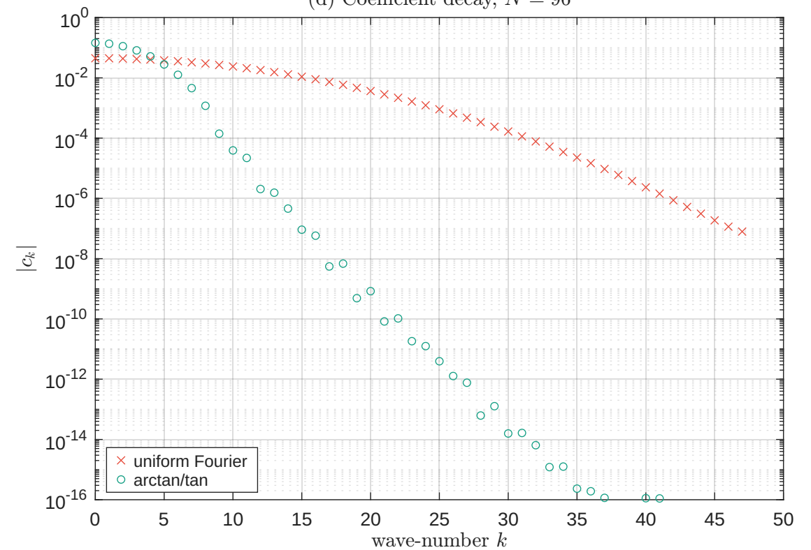
(d) Coefficient decay, N = 96
