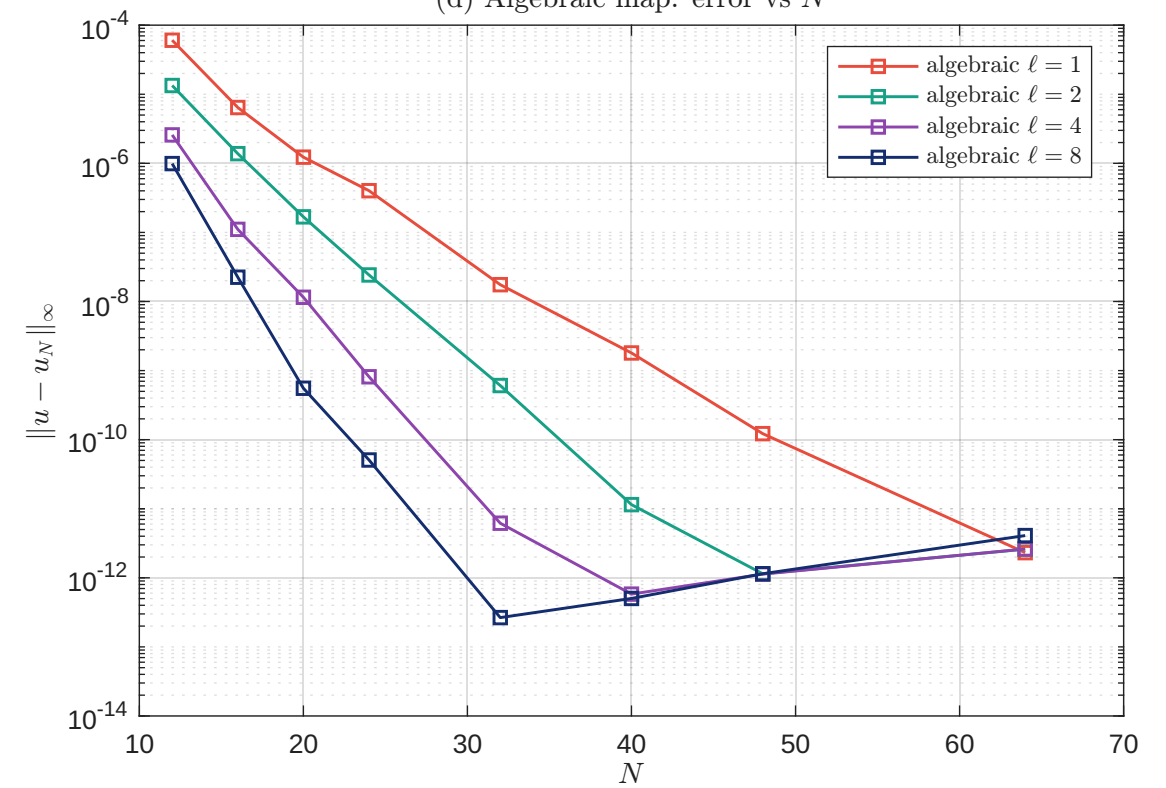
(d) Algebraic map: error vs N
