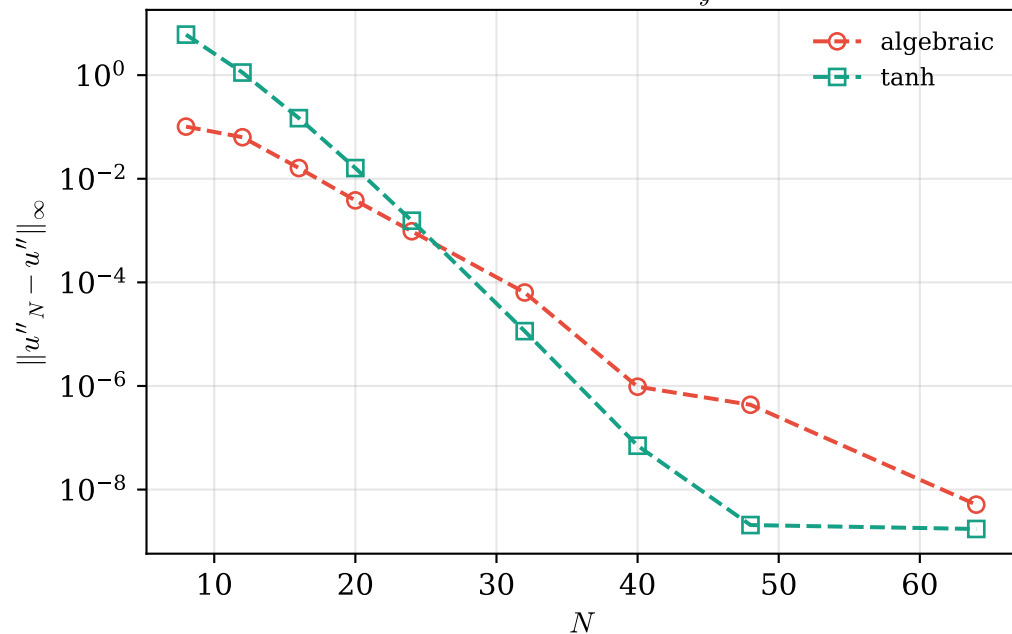
(d) Second derivative: D_y^2 u ( N^2 -lag)
