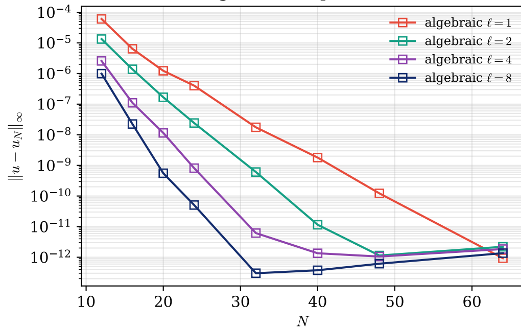
(d) Algebraic map: error vs N
