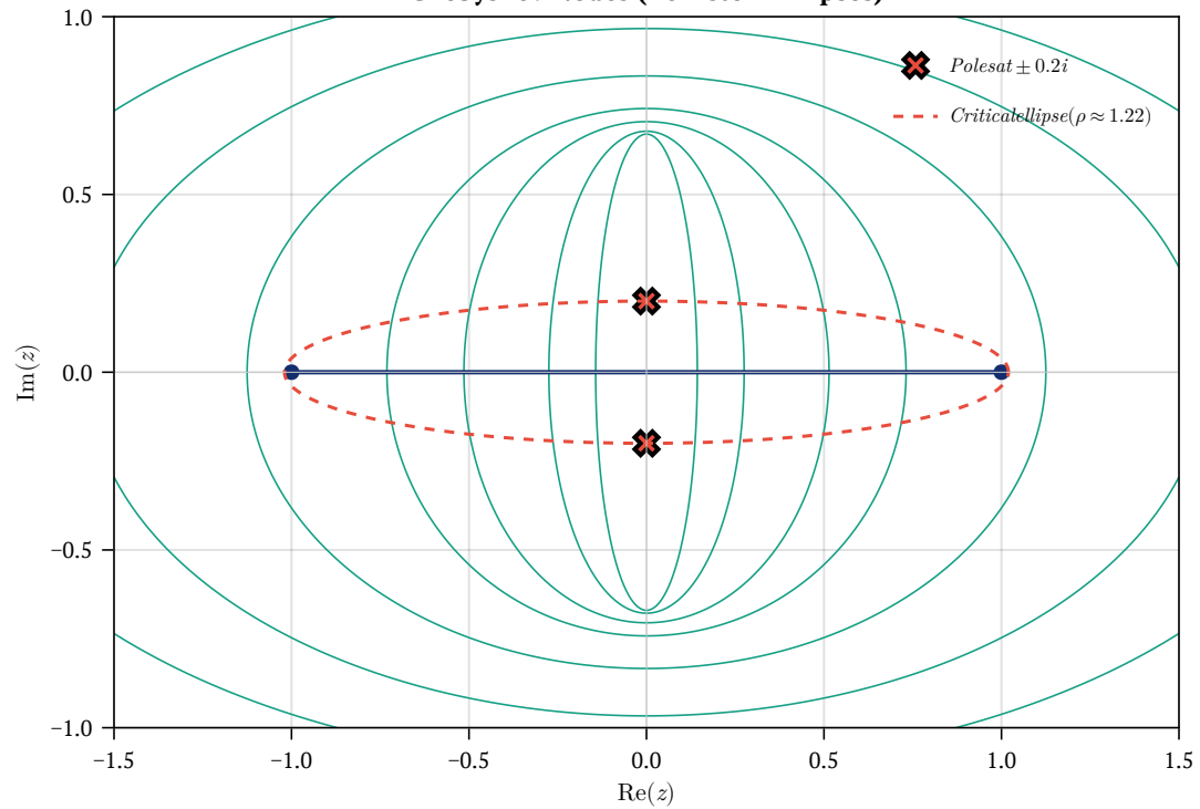
Chebyshev Nodes (Bernstein Ellipses)
