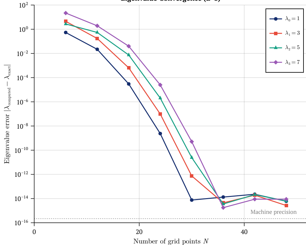
Eigenvalue Convergence (L=8)
