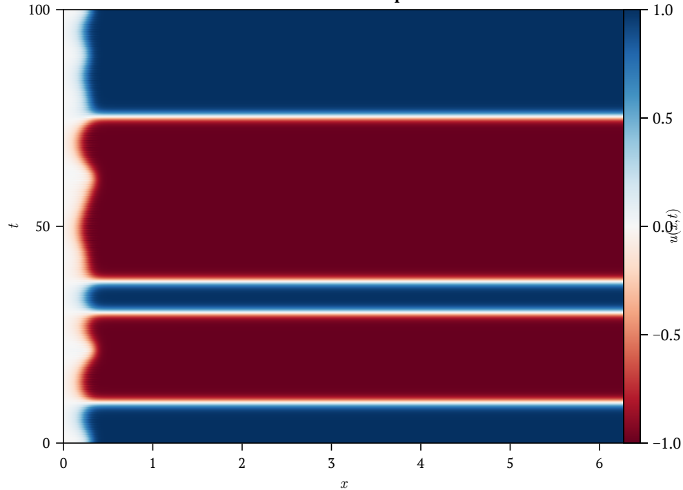
Allen-Cahn: Phase Separation
