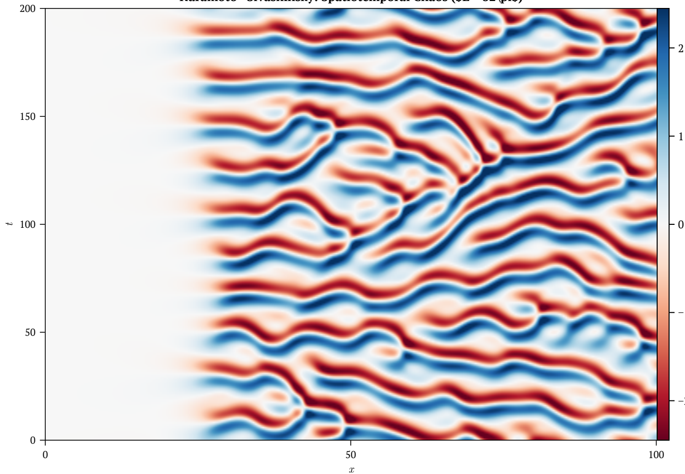
Kuramoto-Sivashinsky: Spatiotemporal Chaos ( L = 32\pi )
