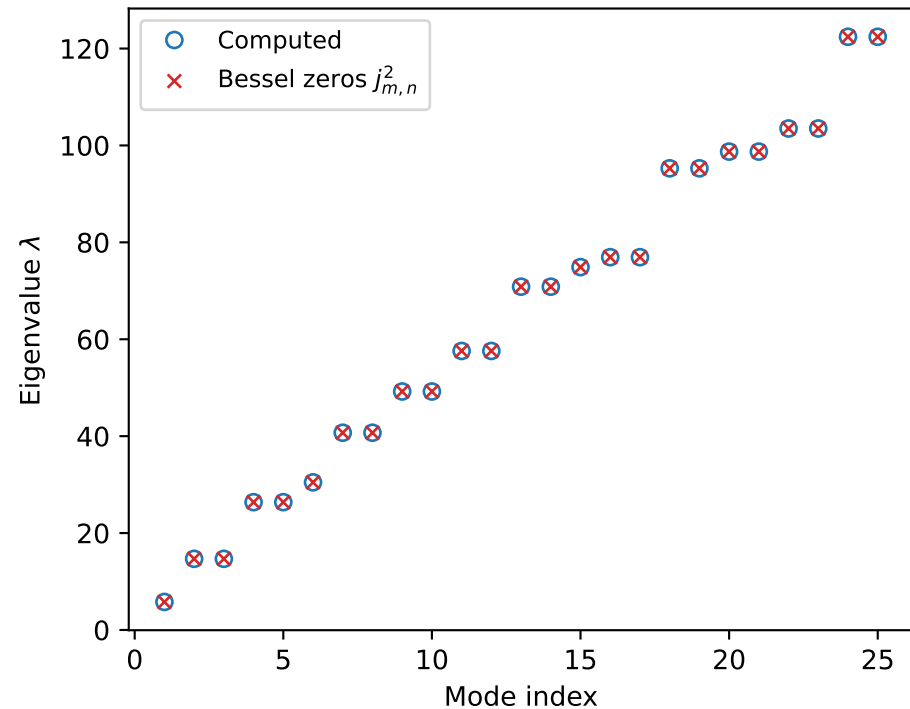
Eigenvalue comparison
