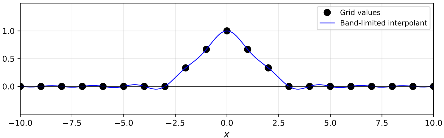
Discrete hat function
