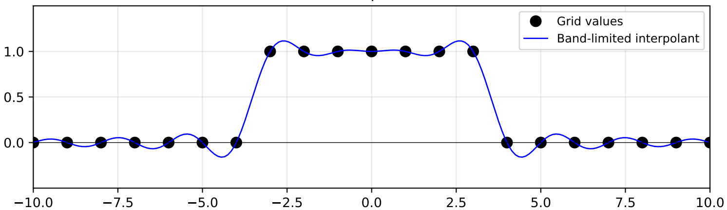
Discrete hat function
