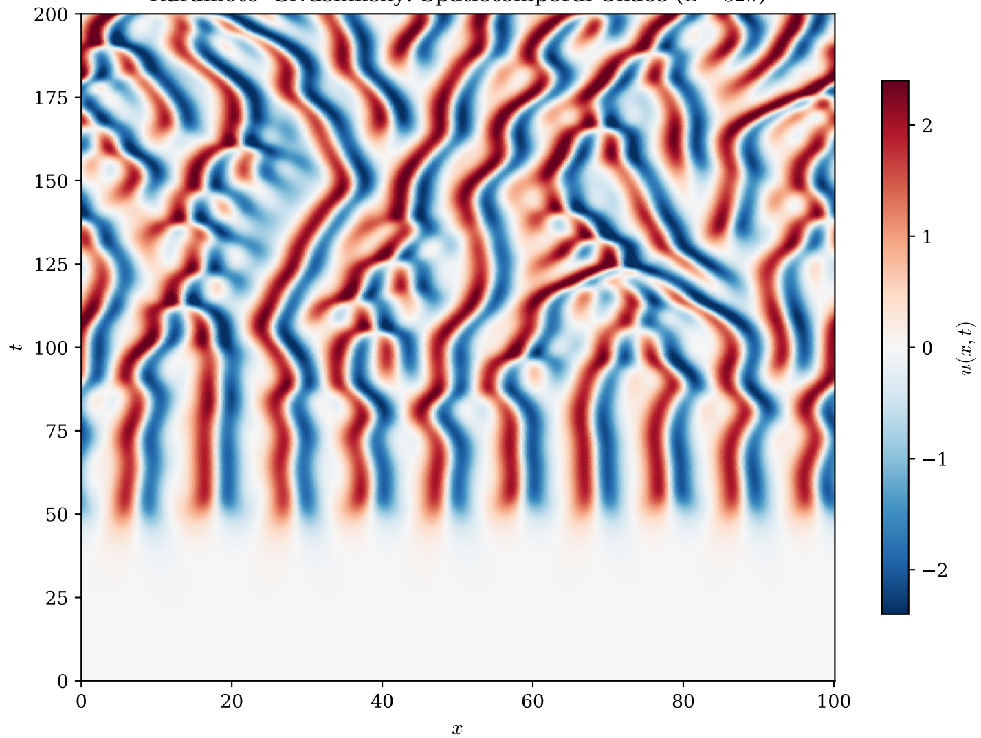
Kuramoto--Sivashinsky: Spatiotemporal Chaos ( L = 32\pi )
