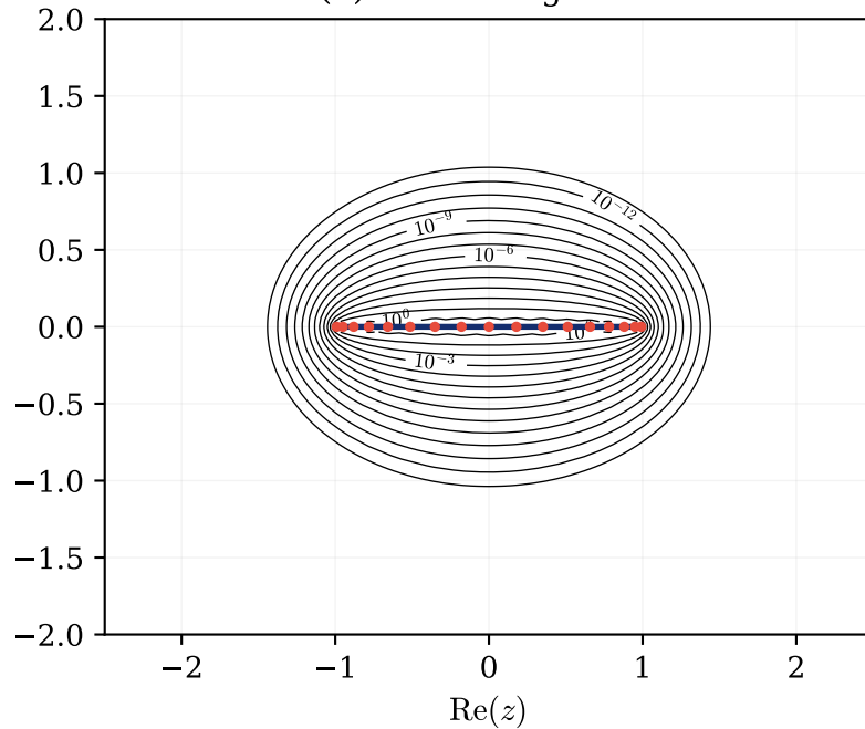
(b) Gauss–Legendre
