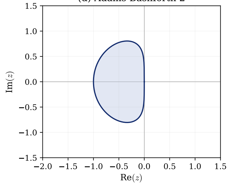
(d) Adams-Bashforth 2
