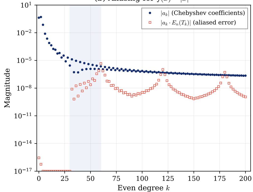
(b) Aliasing for f(x) = |x|^3
