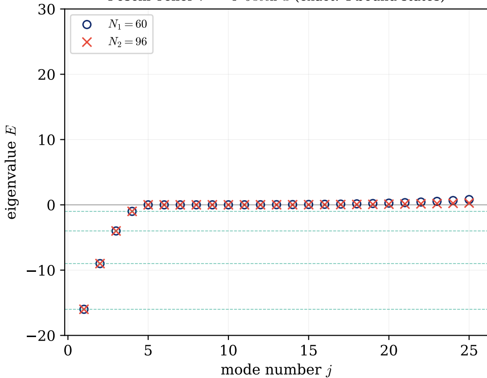
Pöschl-Teller V = -4 \cdot 5 \operatorname{sech}^2 x (exact: 4 bound states)
