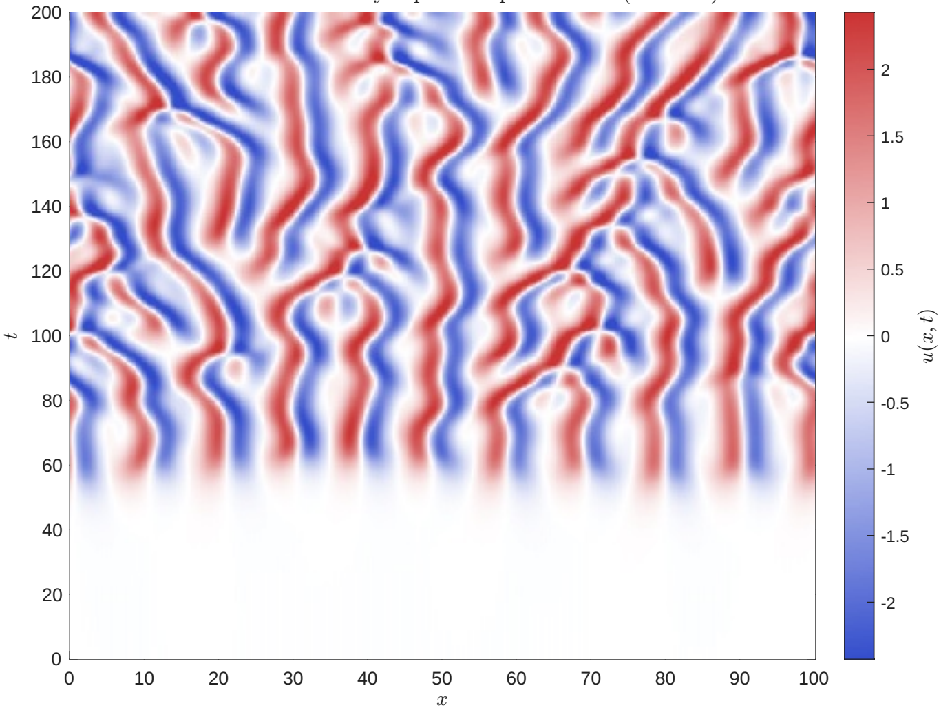
Kuramoto–Sivashinsky: Spatiotemporal Chaos ( L = 32\pi )
