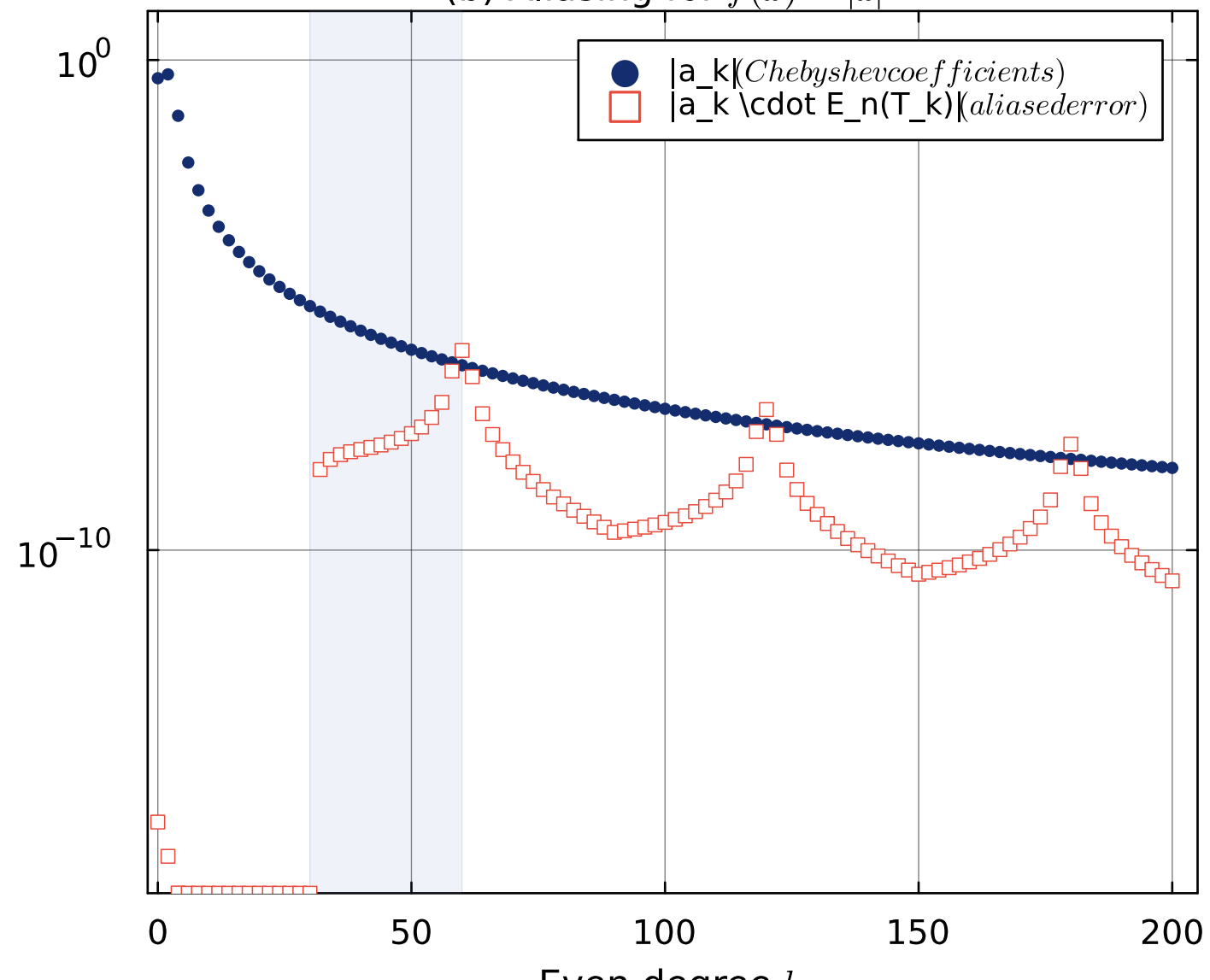
(b) Aliasing for f(x) = |x|^3
