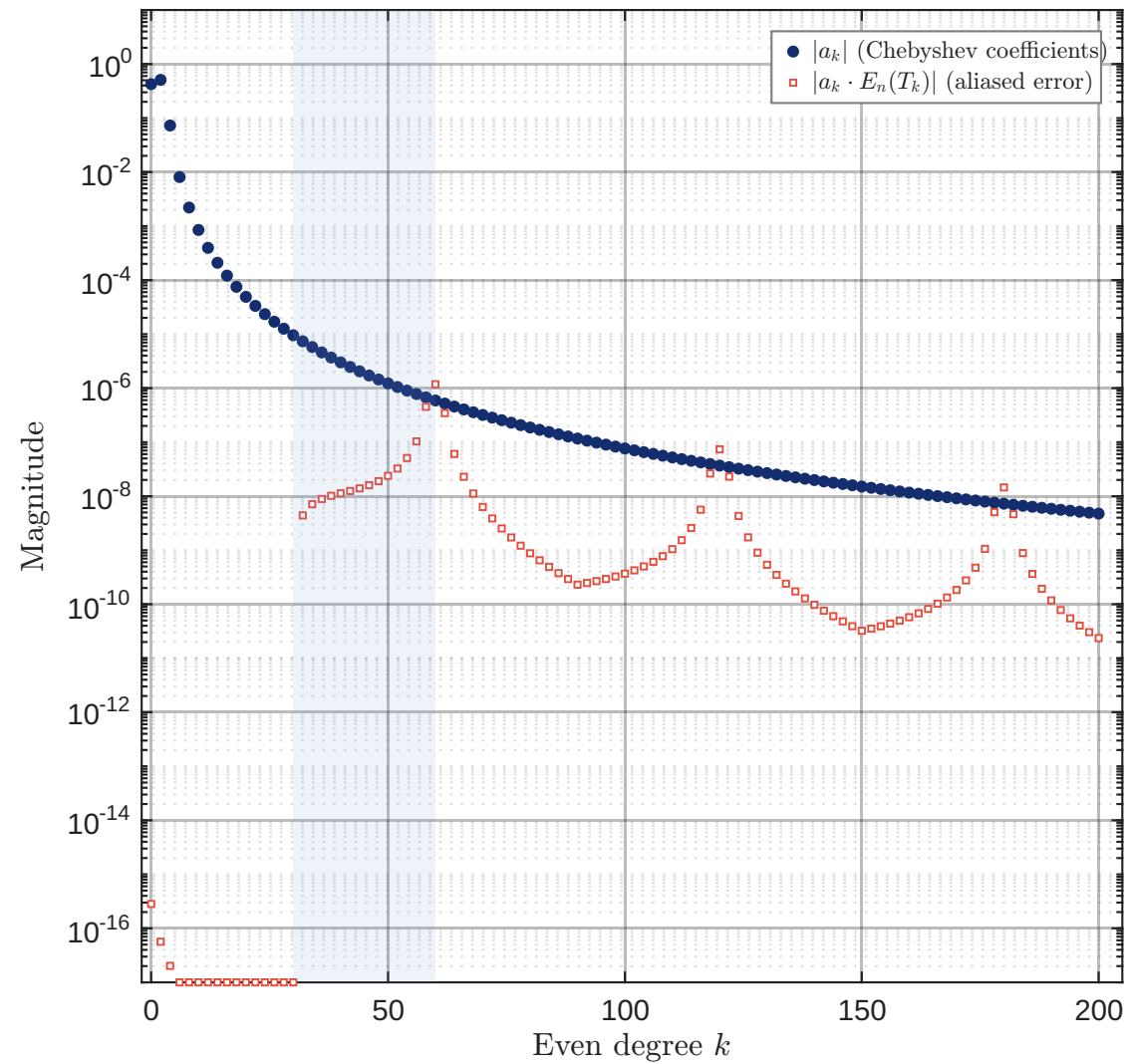
(b) Aliasing for f(x) = |x|^3
