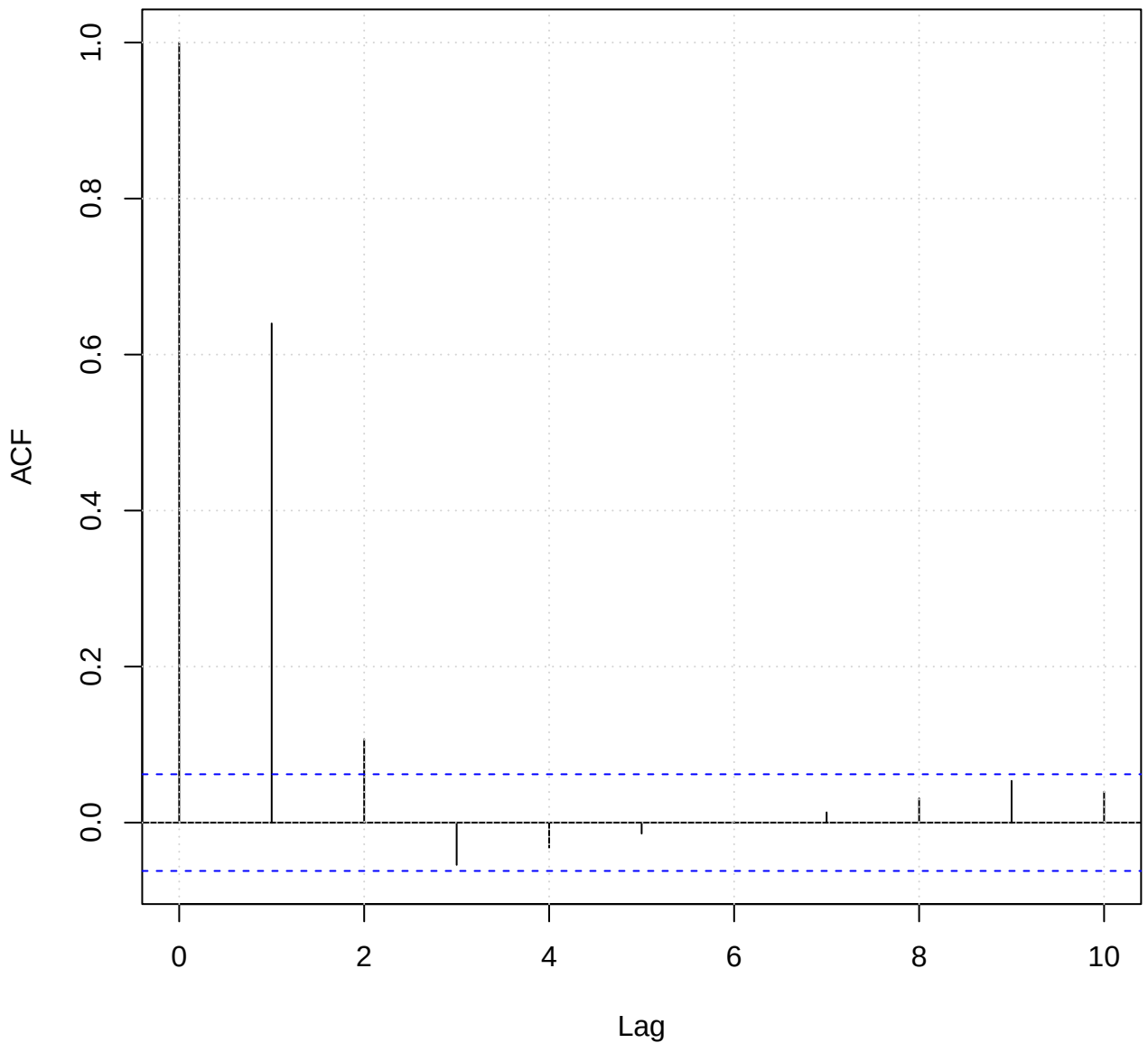
Correlograma del proceso x_t = w_{t-1} + 2w_t + w_{t+1}
